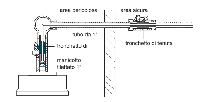
Sensore su tubo da 1" in area con polveri combustibili (per FM, Classe II)
