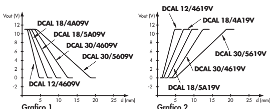
Curve caratteristiche
